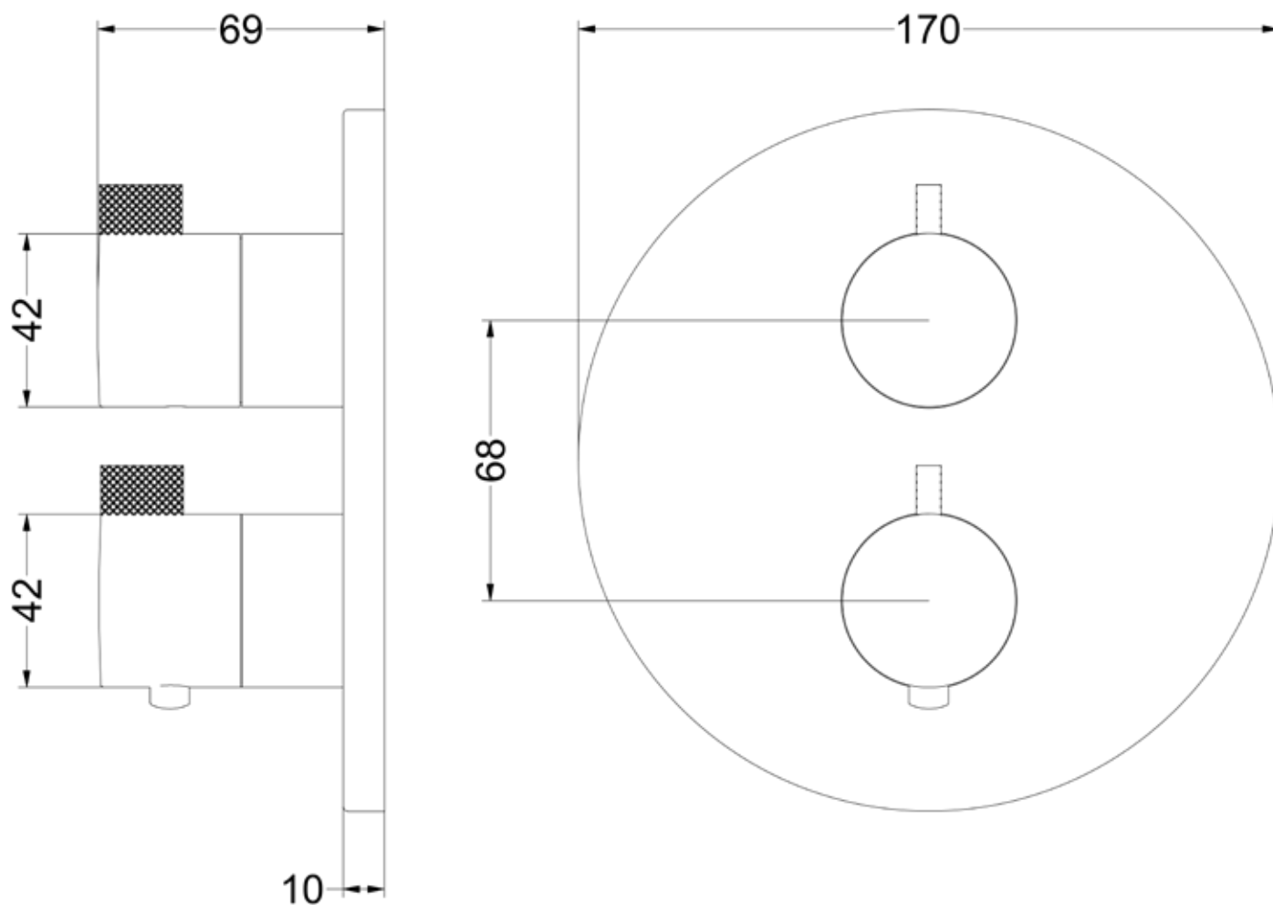
Triba afbouwdeel inbouwthermostaat met 2-weg stop-omstel Triba external part thermostat with 2-way diverter with closing function
