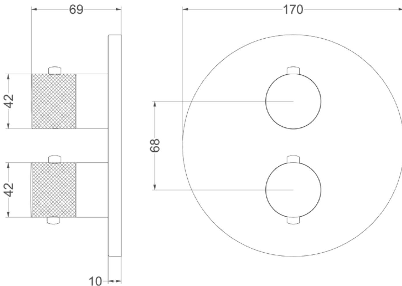
Nexus afbouwdeel inbouwthermostaat met 2-weg stop-omstel Nexus external part thermostat with 2-way diverter with closing function
