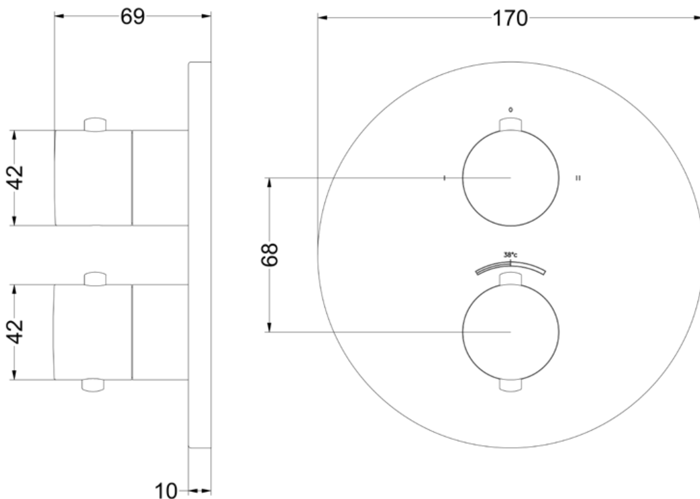
Concord afbouwdeel inbouwthermostaat met 2-weg stop-omstel Concord external part thermostat with 2-way diverter with closing function
