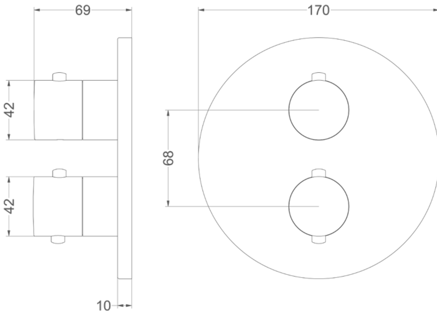
Bond afbouwdeel inbouwthermostaat met 2-weg stop-omstel Bond external part thermostat with 2-way diverter with closing function
