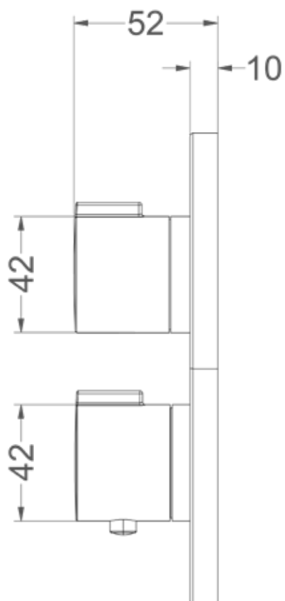
Pact afbouwdeel inbouwthermostaat met 1 losse stopkraan Pact external part of concealed thermostat with 1 stop-diverter
