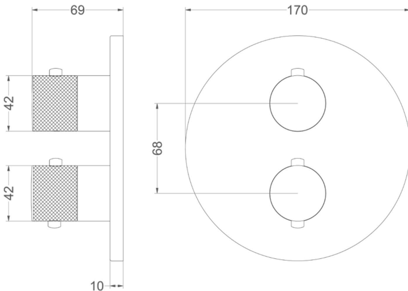
Nexus afbouwdeel inbouwthermostaat met 1 losse stopkraan
