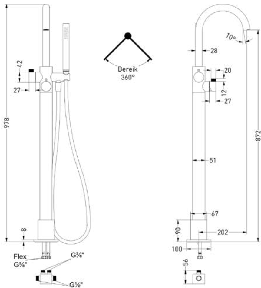
Tribe vrijstaande badmengkraan met staaf handdouche
