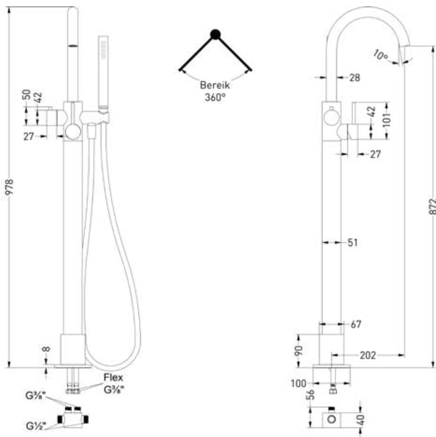
Concord vrijstaande badmengkraan met staaf handdouche
