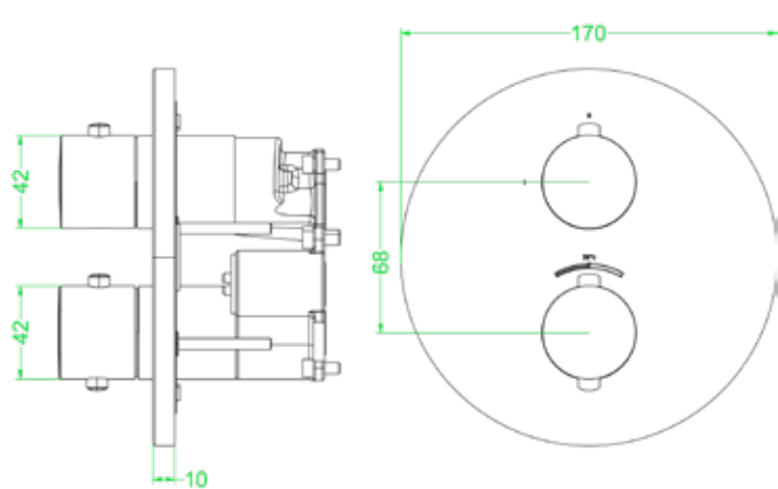
Bond afbouwdeel inbouwthermostaat met 1 losse stopkraan Bond external part of concealed thermostat with 1 stop-diverter
