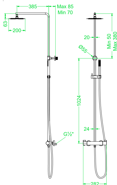
Pact opbouw douche thermostaatkraan met stop-omstel en showerpipe met glijstuk Pact wall-mounted shower thermostatic faucet with stop diverter and shower pipe with sliding piece
