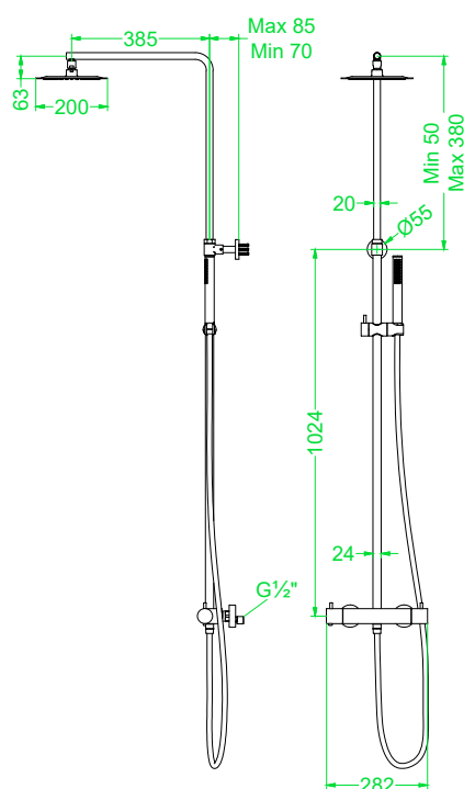
Bond opbouw douche thermostaatkraan met stop-omstel en showerpipe met glijstuk Bond wall-mounted shower thermostatic faucet with stop diverter and shower pipe with sliding piece
