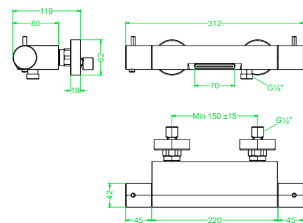
Bond badthermostaat met cascada uitloop Bond bath thermostatic faucet with cascade spout
