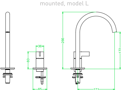
Pact eenhendel wastafelmengkraan, opbouw, 2-gats bladmontage met uitloop
