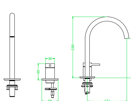
Bond eenhendel wastafelmengkraan, opbouw, 2-gats bladmontage met uitloop
