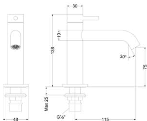
Bond staand S
