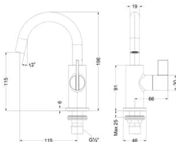
Pact met draaibare uitloop Pact deck mounted with swivel spout
