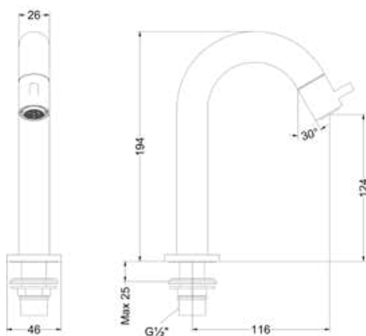
Bond staand gebogen S
