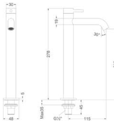
Bond staand L
