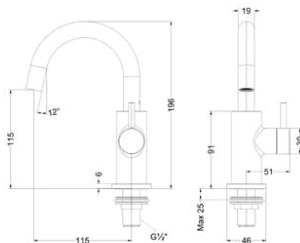
Bond met draaibare uitloop
