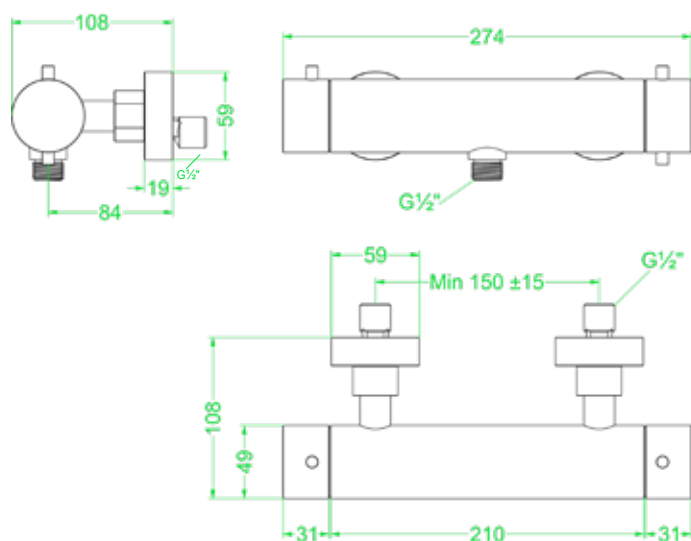
Concord douchethermostaatkraan opbouw
