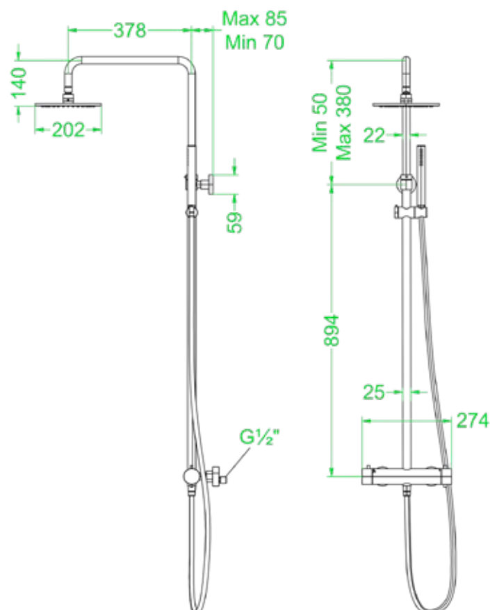
Concord opbouw douche thermostaatkraan met stop-omstel en glijstang met glijstuk (combiset 1)
