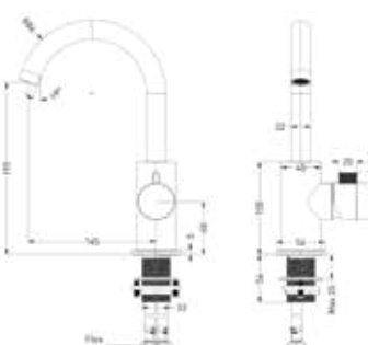
Tribe eenhendel wastafelmengkraan, opbouw, met draaibare uitloop
