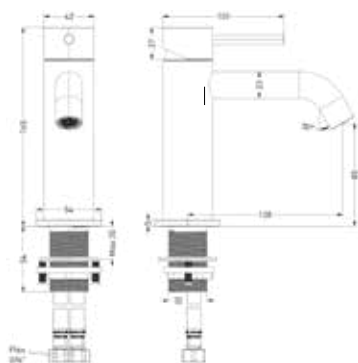
Concord eenhendel wastafelmengkraan, opbouw, model S
