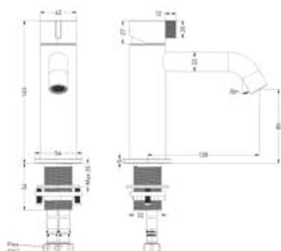
Tribe eenhendel wastafelmengkraan, opbouw, model S
