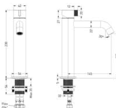
Tribe eenhendel wastafelmengkraan, opbouw, model M
