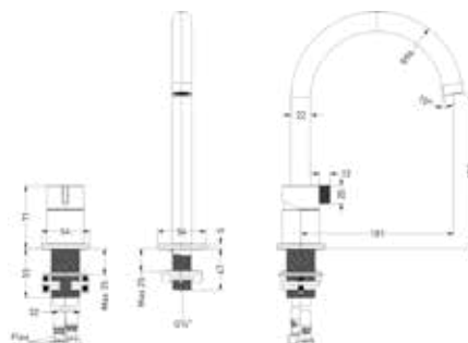
Tribe eenhendel wastafelmengkraan, opbouw, 2-gats bladmontage met uitloop
