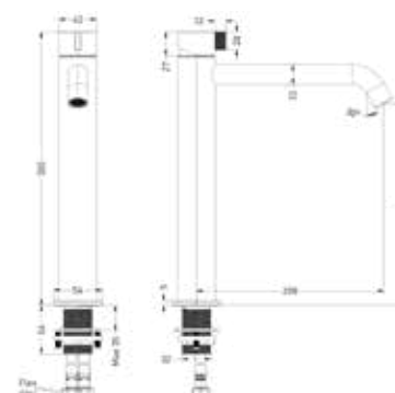
Tribe eenhendel wastafelmengkraan, opbouw, model L
