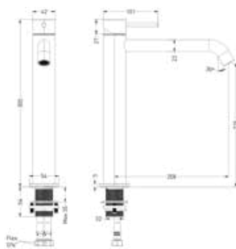
Concord eenhendel wastafelmengkraan, opbouw, model L
