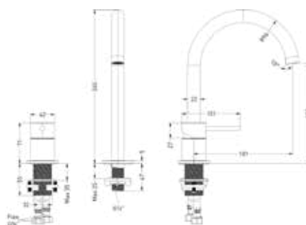
Concord eenhendel wastafelmengkraan, opbouw, 2-gats bladmontage met uitloop
