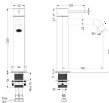
Concord eenhendel wastafelmengkraan, opbouw, model M
