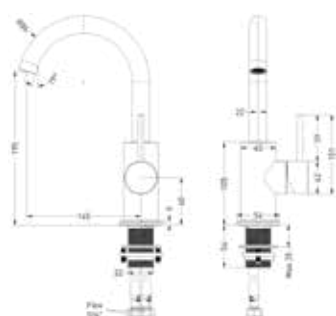
Concord eenhendel wastafelmengkraan, opbouw, met draaibare uitloop
